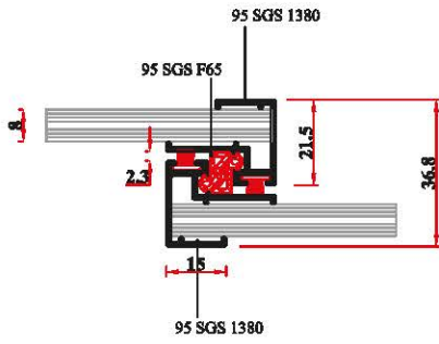
2 NOLU DETAY
