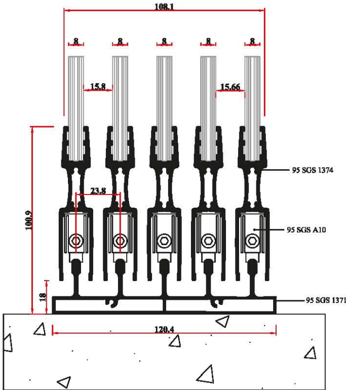
2 NOLU DETAY
