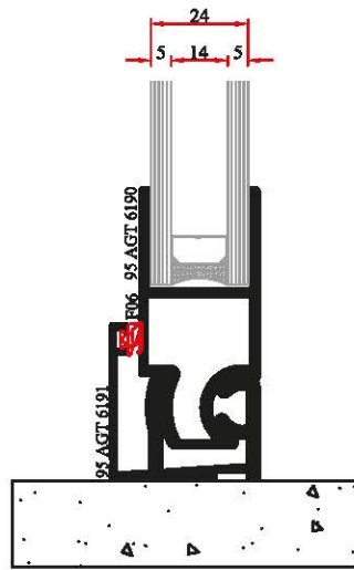
Silinebilir Alt Profil Detayı
