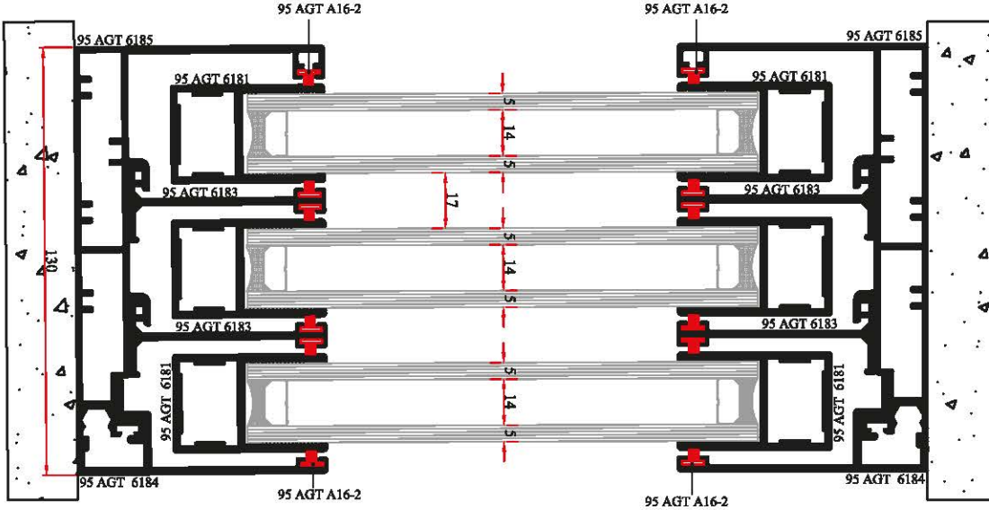
Düz Yan Dikme Kesiti
