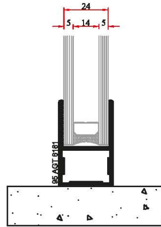
Düz Alt Profil Detayı
