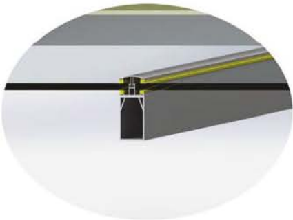
ORTA TAŞIYICI DETAYI
